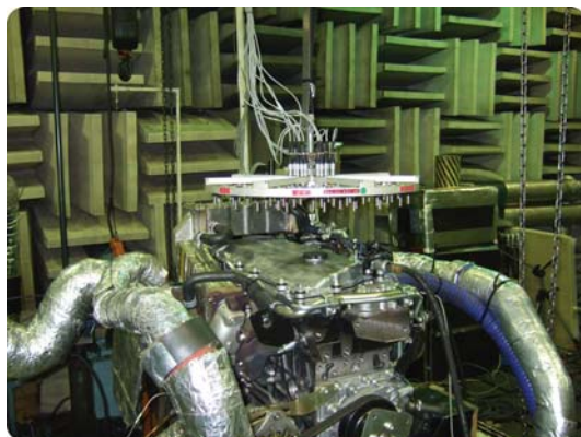
Fig. 2 84 チャンネルのセクターホイールアレイを使用し、エンジン A とエンジン B を対象として半無響室で行われた SONAH（左）およびビームフォーミング（右）の測定
