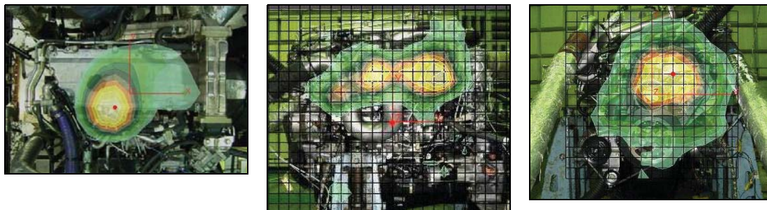
Fig. 4 ビームフォーミングによる 様々なメトリクスのマッ ピング：左から、定常ラウド ネス、ラフネス、結合メ トリクス
