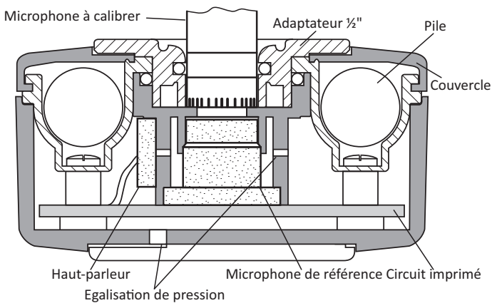
Fig. 1 Vue en coupe du Calibreur acoustique Type 4231. Le circuit d'asservissement intègre un microphone à condensateur de haute qualité assurant la stabilité du niveau de pression acoustique
