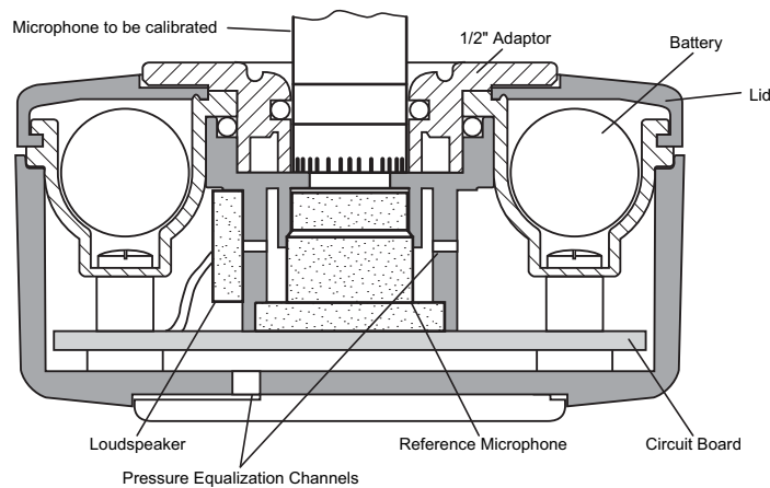
Fig. 1 Sezione trasversale del calibratore di livello sonoro tipo 4231. Il ciclo di reazione si basa su un microfono condensatore di alta qualità che assicura un livello di pressione sonora molto stabile
